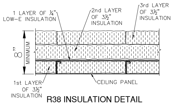
'S' TYPE BLDG.
